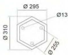
TRỤ 302 L800 x H4000 E27 x 3 17.500.000đ
