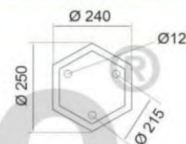
CHÂN ĐẾ 13 H630 - Nhôm 3.050.000đ
