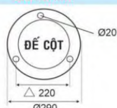
CHÂN ĐẾ 04 H700 - Gang 5.650.000đ
