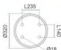
CHÂN ĐẾ 15 H1180 - Nhôm 9.900.000đ
