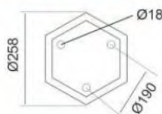
CHÂN ĐẾ 01 H450 - Gang 2.750.000đ
